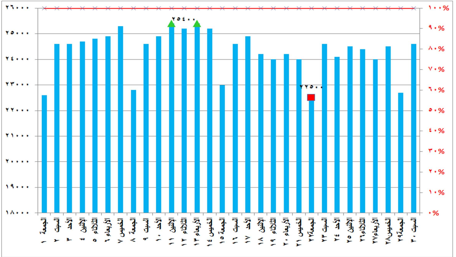
شكل (٥) قدرات الانتاج المتاحة ونسبتها للحمل الأقصى خلال شهر نوفمبر ٢٠١٩
