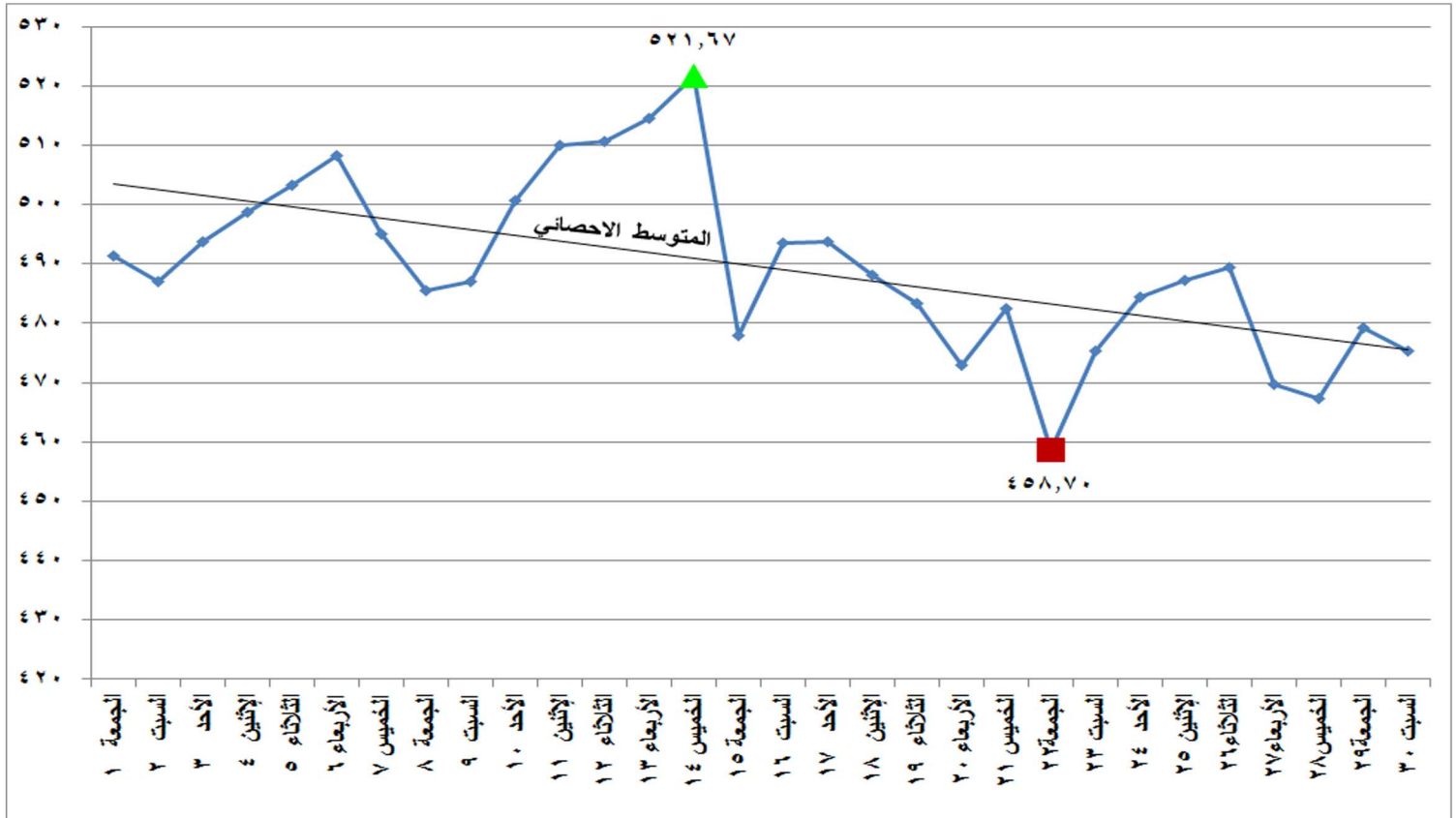
شكل (١٥) إجمالي الطاقة الكهربائية المنتجة من كل المصادر الأولية خلال شهر نوفمبر ٢٠١٩
