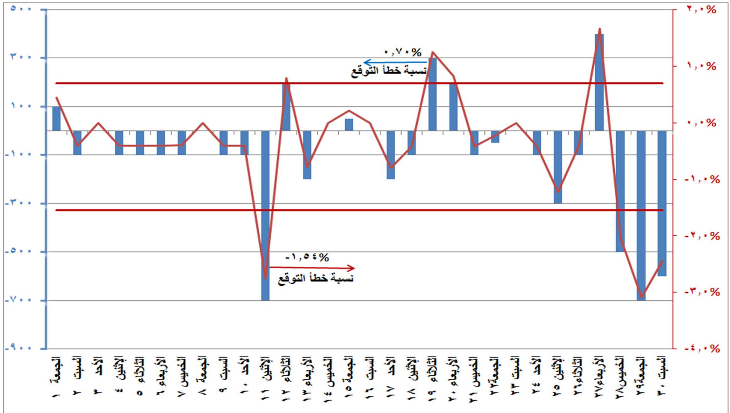
شكل (١٠) الفرق بين الحمل الأقصى المتوقع والمسجل فعليا ونسبة الفرق إلى الحمل المسجل فعليا خلال شهر نوفمبر ٢٠١٩
