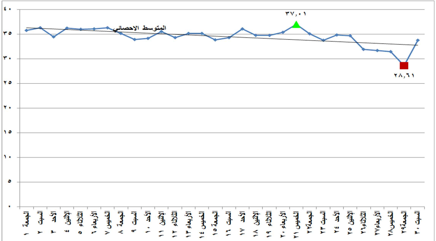
شكل (٢٣) الطاقة الكهربائية المنتجة من المصادر المائية خلال شهر نوفمبر ٢٠١٩
