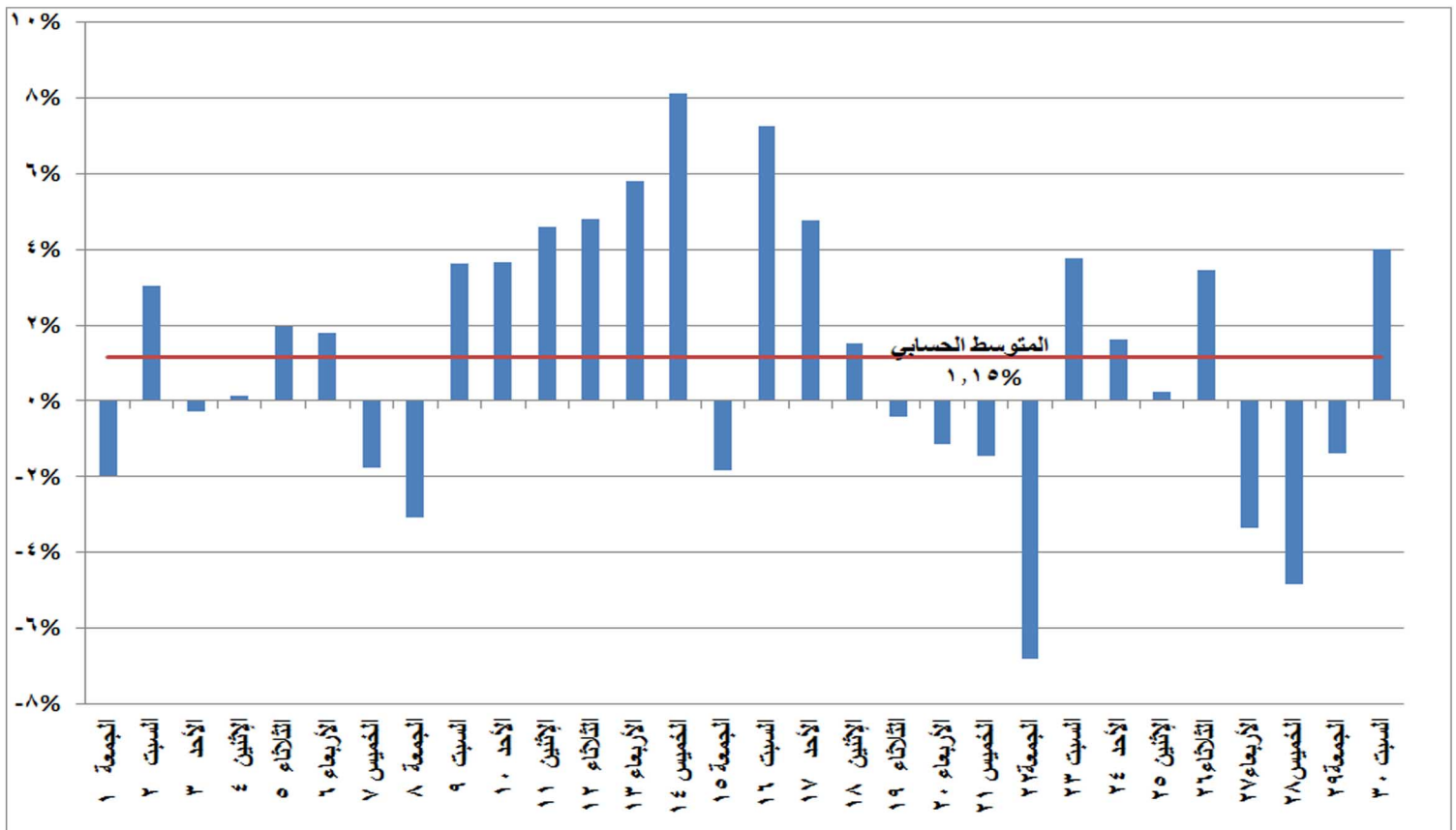
شكل (١٦) نسب التغير في الطاقة الكهربائية المنتجة خلال شهر نوفمبر ٢٠١٩ مقارنة بالشهر المماثل من العام السابق
