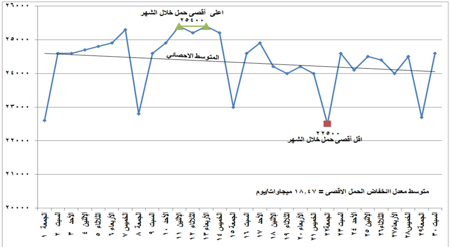
شكل (١) تطور الحمل الاقصى اليومي خلال شهر نوفمبر ٢٠١٩
