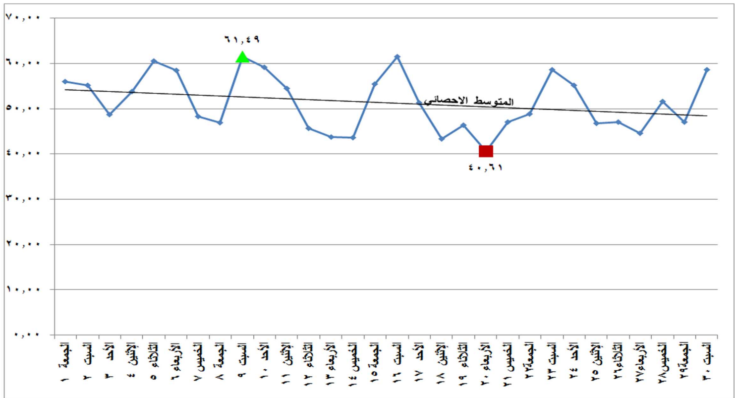
شكل (٢١) الطاقة الكهربائية المنتجة من المصادر غير الحرارية خلال شهر نوفمبر ٢٠١٩
