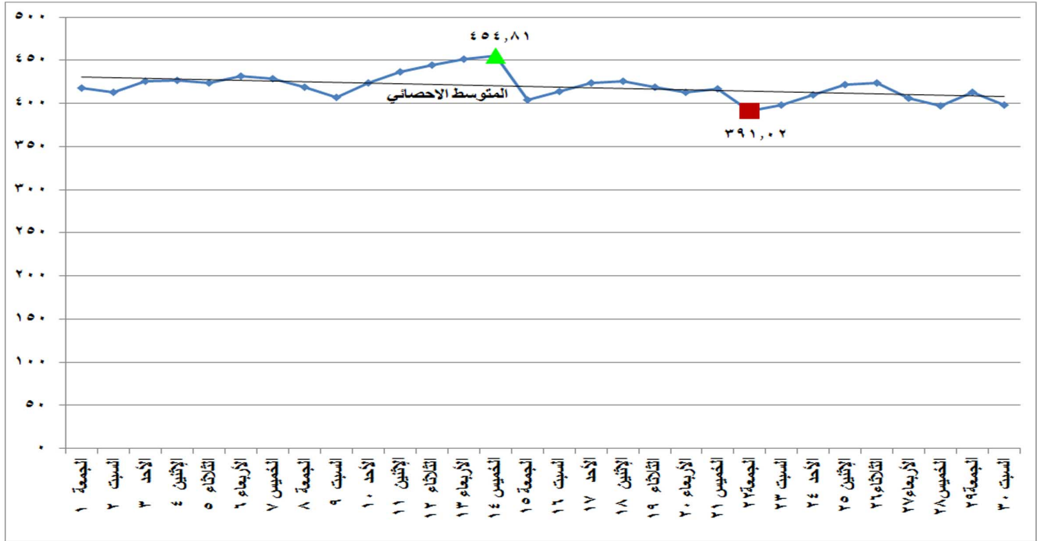
شكل (١٧) الطاقة الكهربائية المنتجة من الغاز الطبيعي خلال شهر نوفمبر ٢٠١٩
