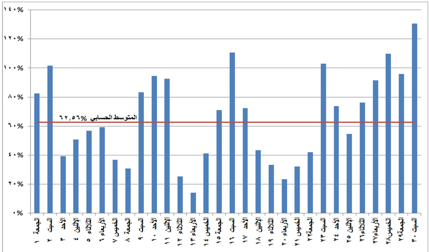
شكل (٢٢) نسب التغير في استخدام المصادر غير الحرارية في إنتاج الطاقة الكهربائية خلال شهر نوفمبر ٢٠١٩ مقارنة بالشهر المماثل من العام السابق
