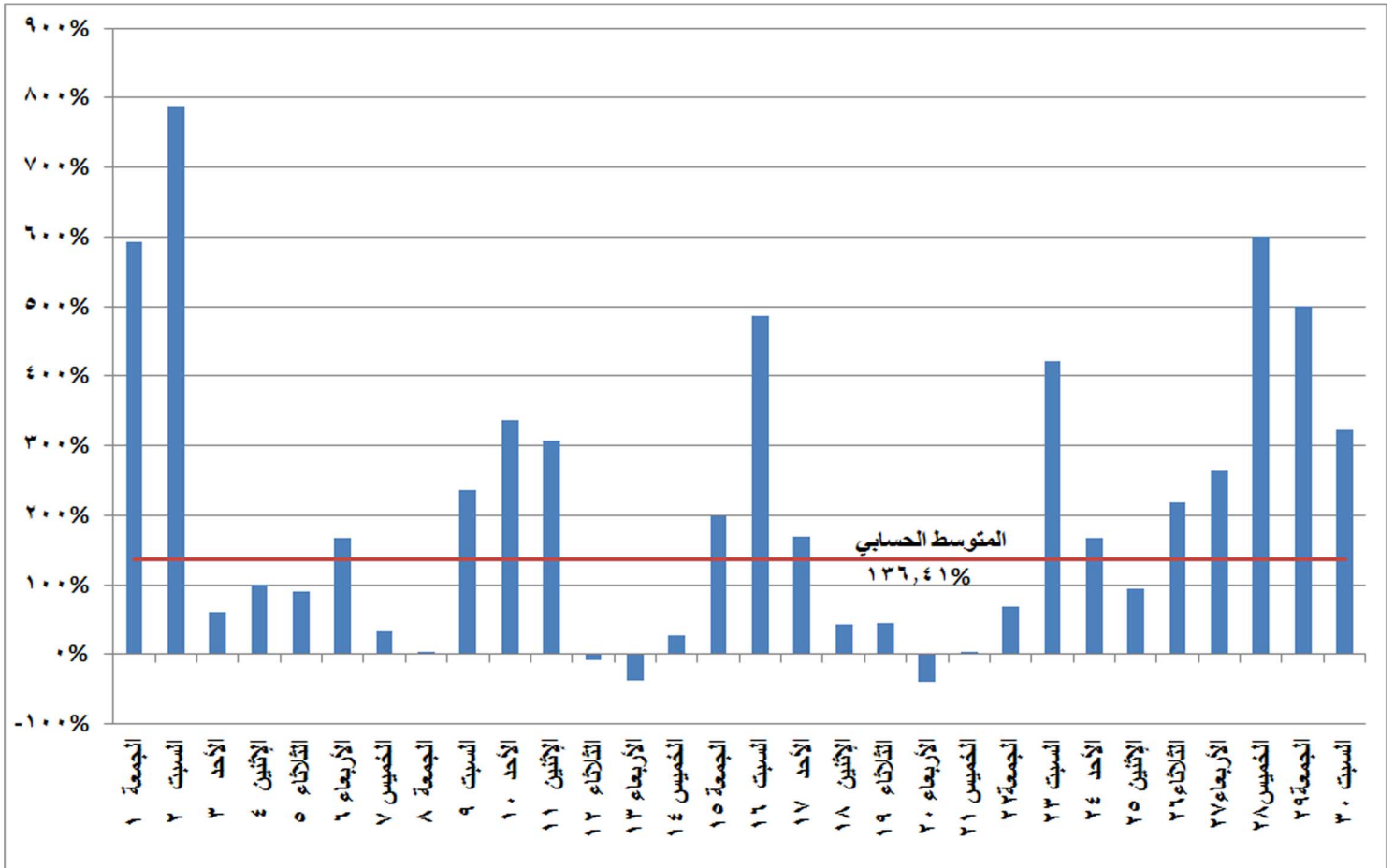
شكل (٢٦) نسب التغير في استخدام الرياح والشمس في إنتاج الطاقة الكهربائية خلال شهر نوفمبر ٢٠١٩ مقارنة بالشهر المماثل من العام السابق
