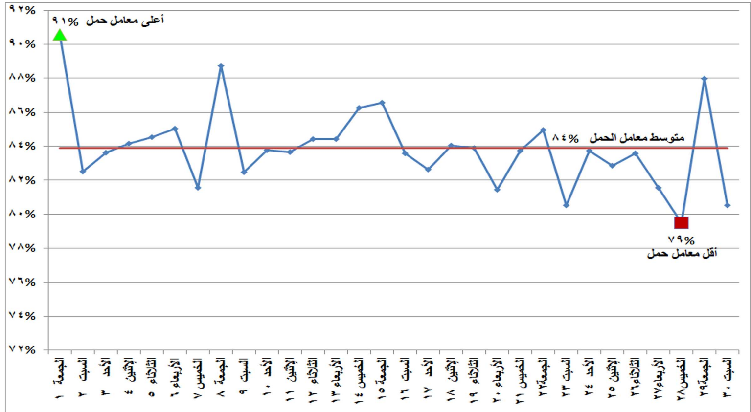
شكل (١٢) إجمالي معامل الحمل لوحدات الانتاج خلال شهر نوفمبر ٢٠١٩
