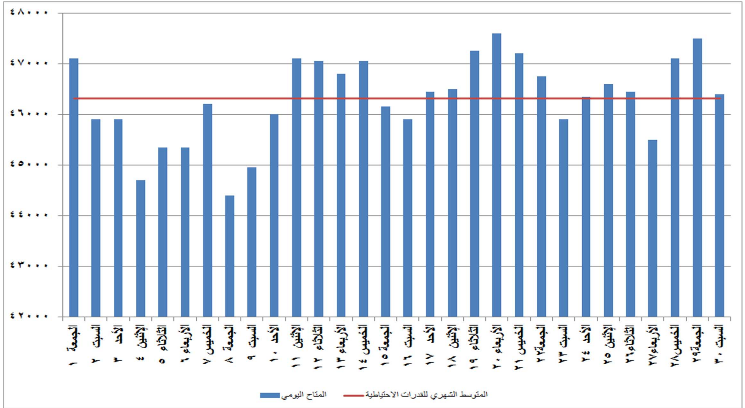
شكل (٢٧) القدرات المتاحة يوميا والمتوسط الشهري للقدرة الاحتياطية خلال شهر نوفمبر ٢٠١٩
