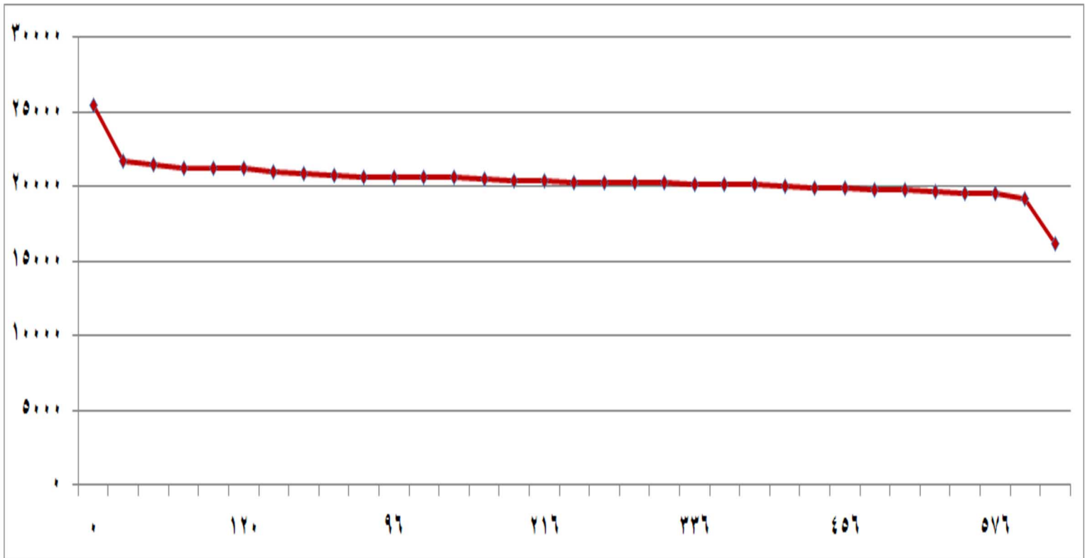
شكل (٨) المنحنى الشهري لفترة الحمل نوفمبر ٢٠١٩
