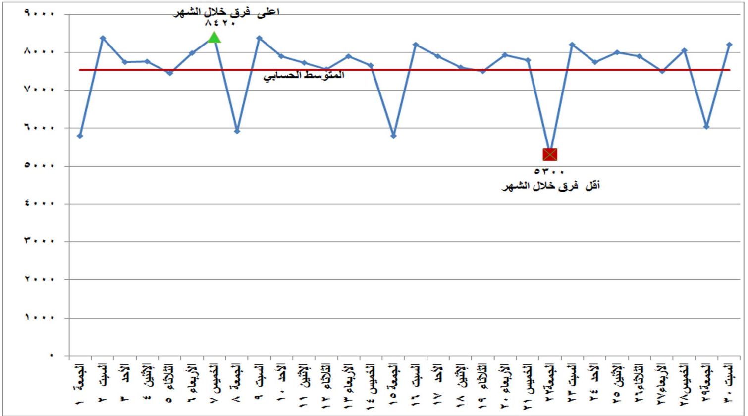
شكل (٣) الفرق بين أقصى وأدنى حمل خلال شهر نوفمبر ٢٠١٩
