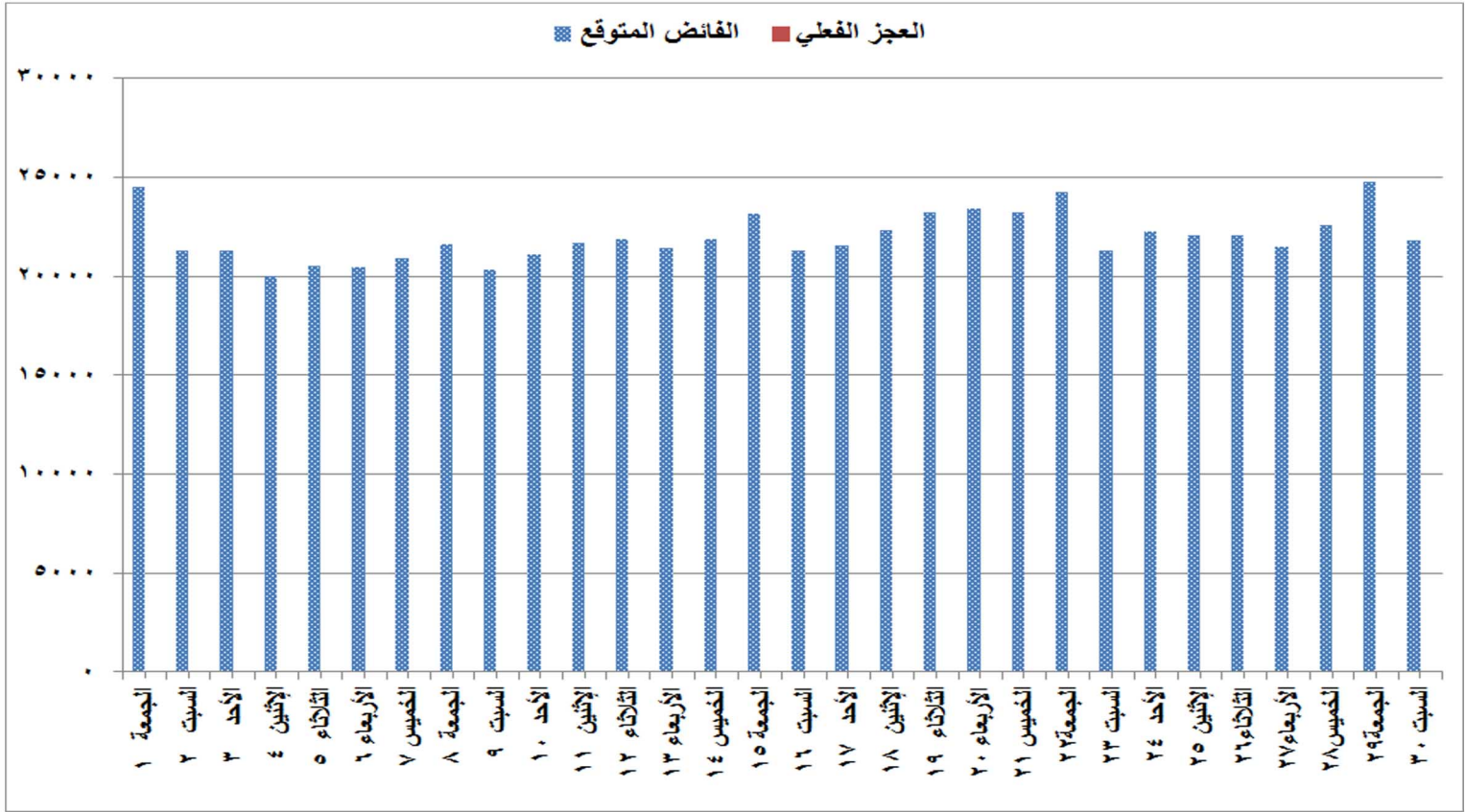
شكل (٧) الفائض والعجز المتوقع للقدرات خلال شهر نوفمبر ٢٠١٩
