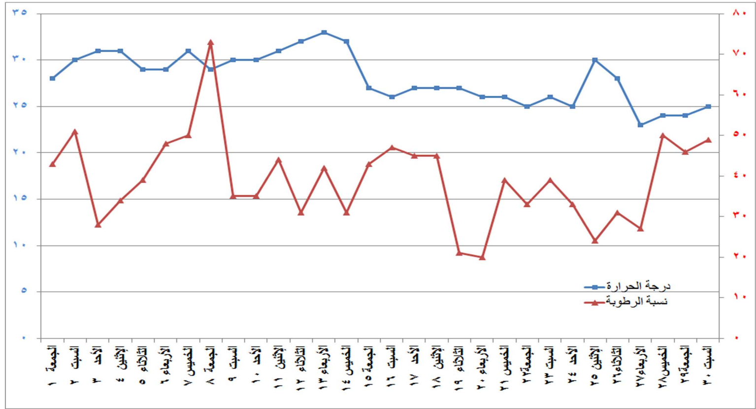
شكل (١١) التغيير في درجة الحرارة والرطوبة النسبية خلال شهر نوفمبر ٢٠١٩
