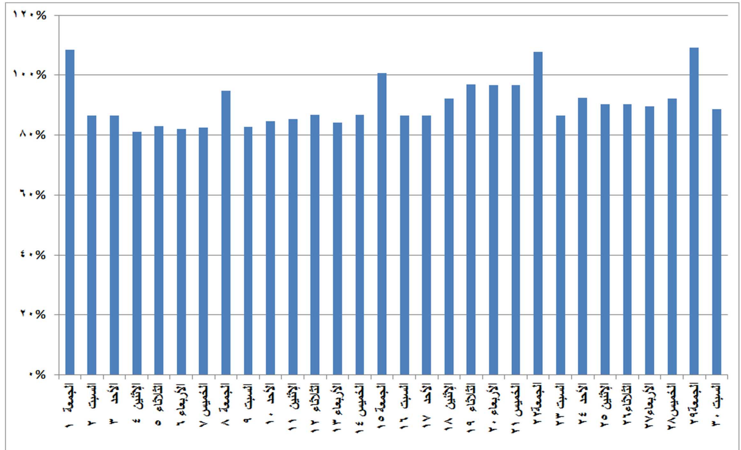
شكل (٢٨) نسب الفائض للحمل الاقصى المسجل يوميا خلال شهر نوفمبر ٢٠١٩
