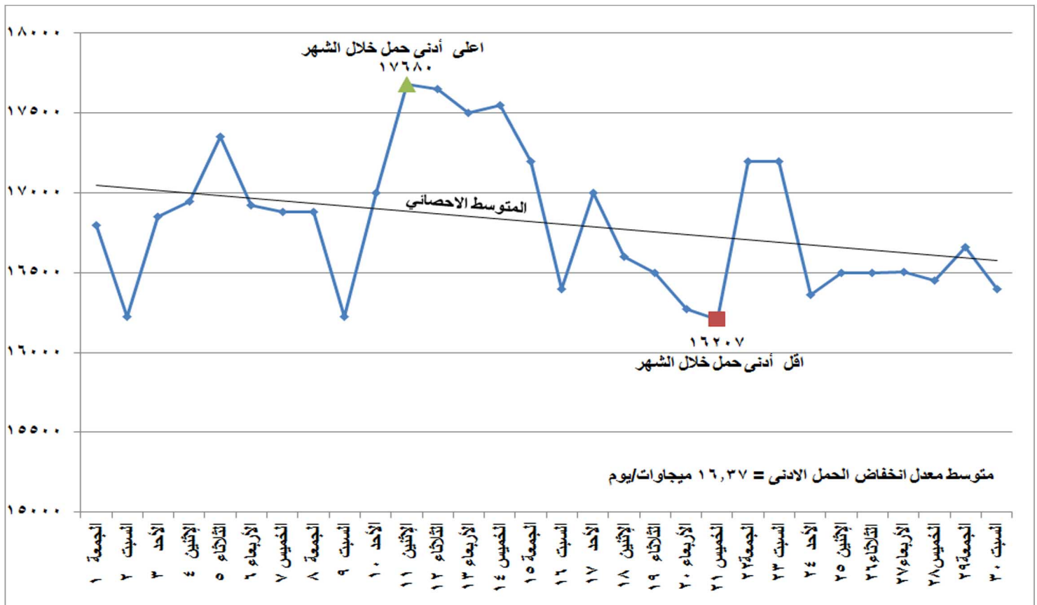
شكل (٢) تطور الحمل الادنى اليومي خلال شهر نوفمبر ٢٠١٩
