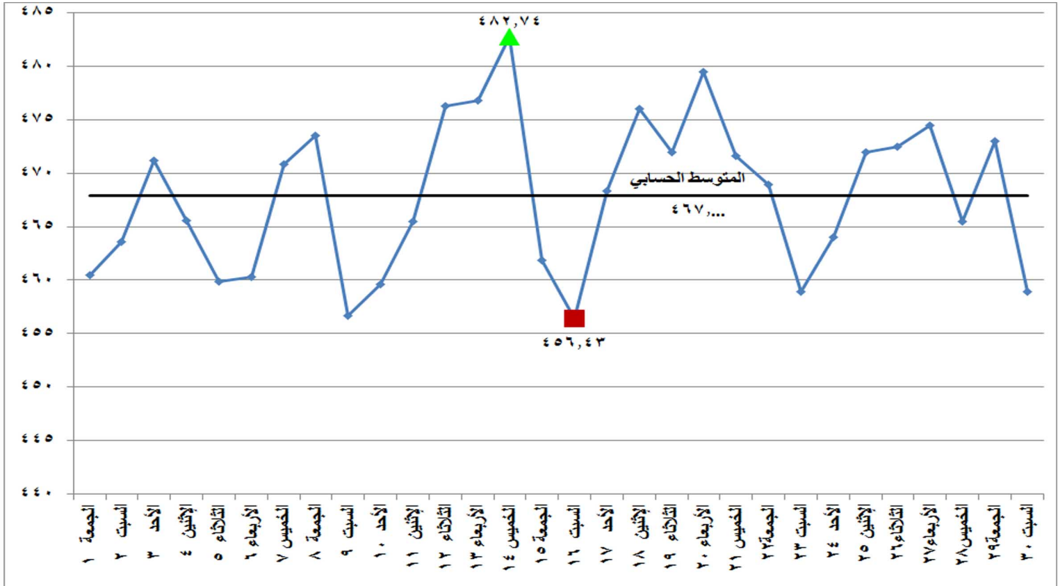
شكل (١٤) معامل انبعاثات غاز ثاني اكسيد الكربون المكافئ على مدى شهر نوفمبر ٢٠١٩
