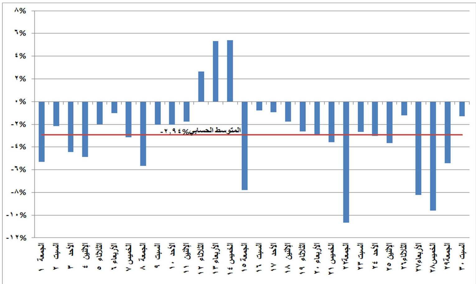
شكل (١٨) نسب التغير في استخدام الغاز الطبيعي في إنتاج الطاقة الكهربائية خلال شهر نوفمبر ٢٠١٩ مقارنة بالشهر المماثل من العام السابق
